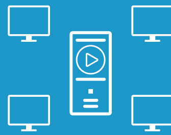
Клиент/сервер
